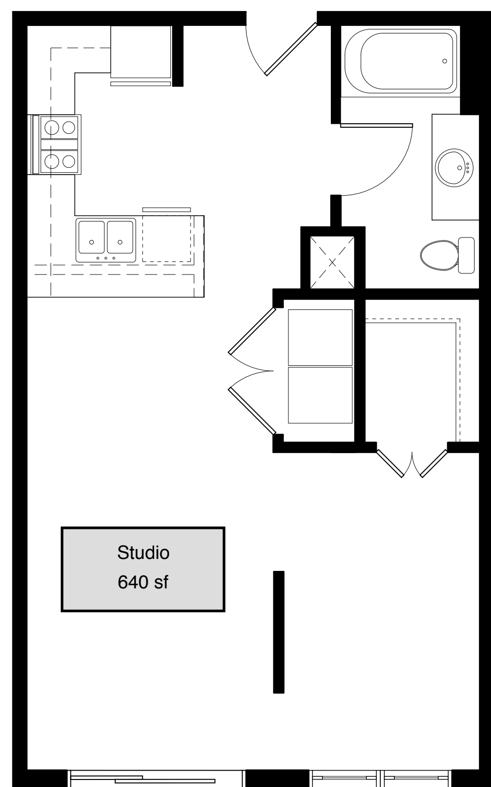
1 STUDIO UNIT A-101 SCALE: 1/4" = 1'-0"
